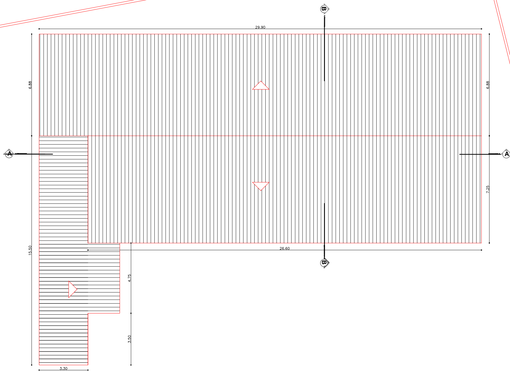
PLANTA DE COBERTA ESCALA 1/100
